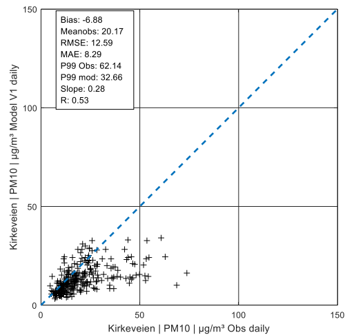
Figure A 120: Daily values PM 10 in Kirkeveien, V1
