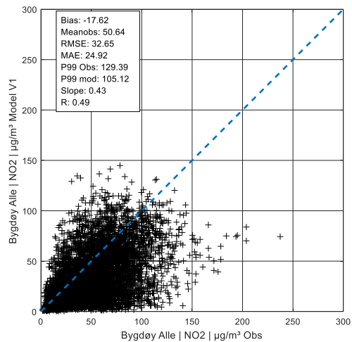
Figure A 86: Yearly value NO 2 in Bygdøy, V1
