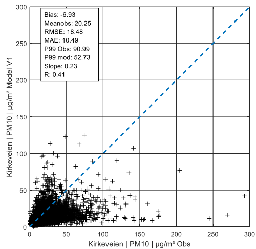
Figure A 119: Hourly values PM 10 in Kirkeveien, V1
