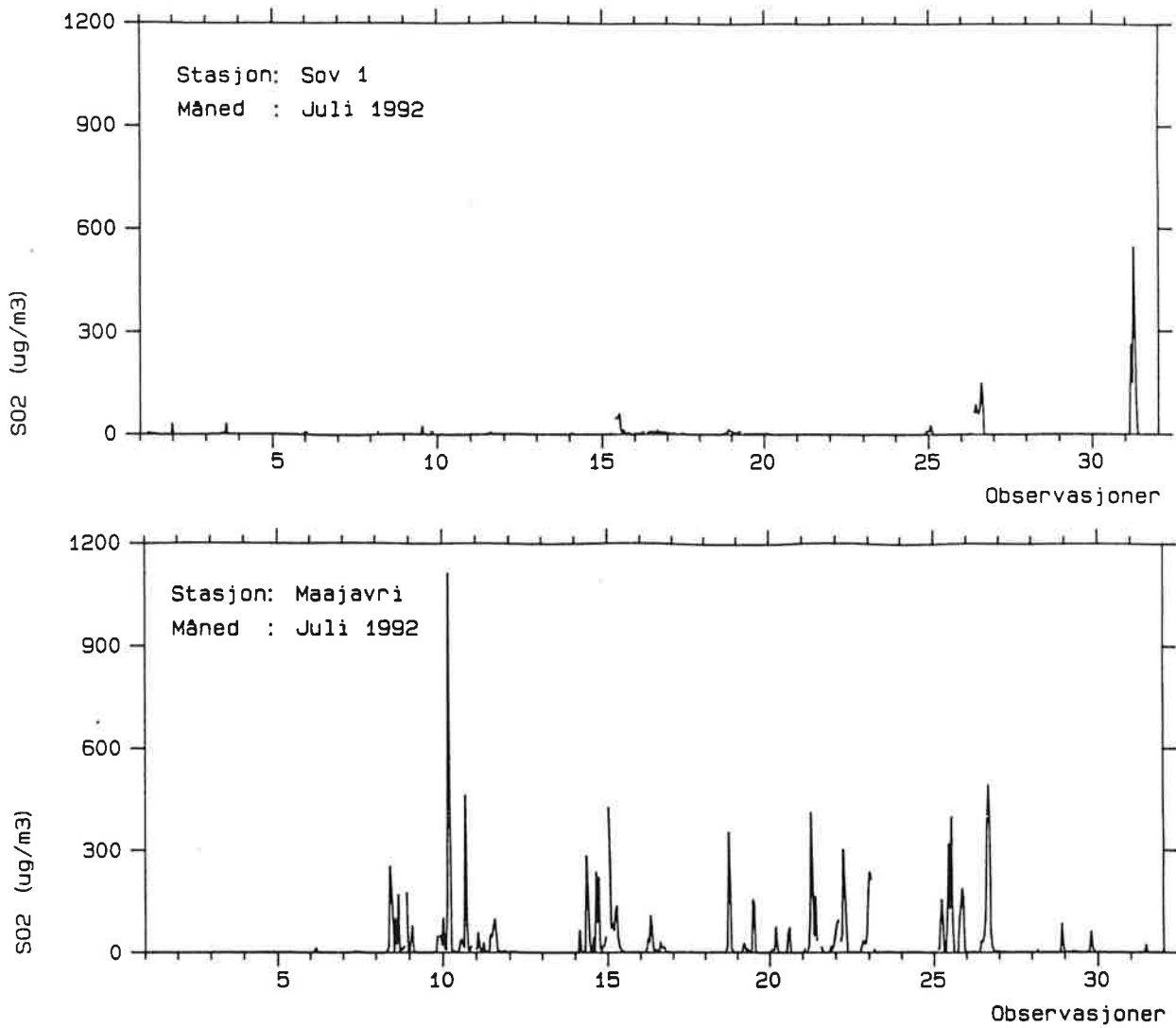
Figur 20: Timemiddelkonsentrasjoner av SO_2 i juli 1992 på SOV 1 og Maajavri ( \mu\text{g}/\text{m}^3 ).
