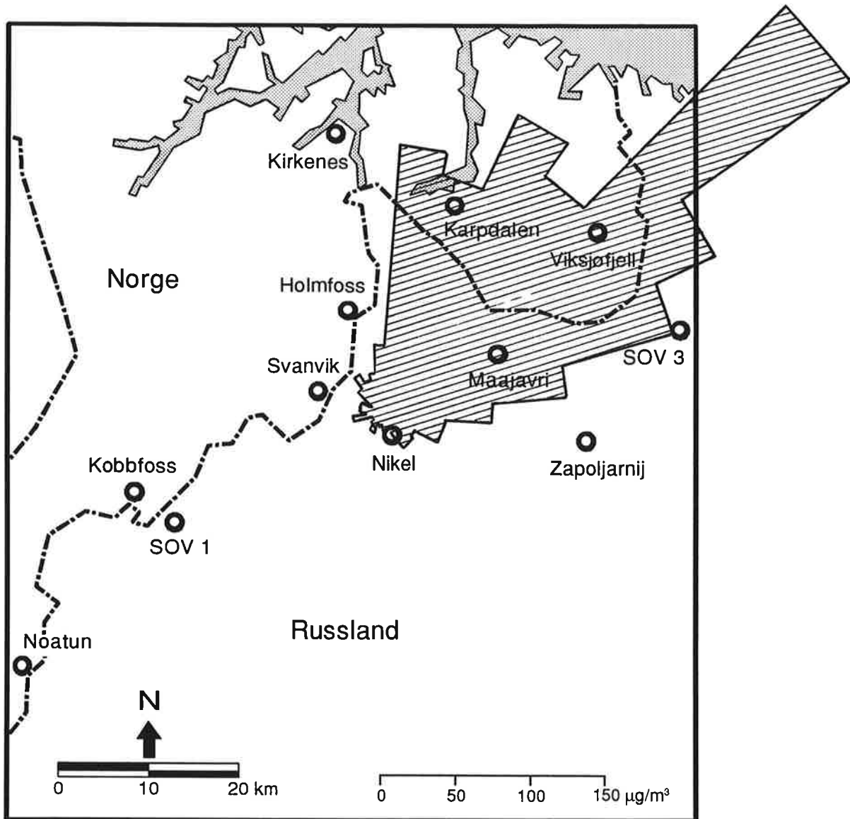
Figur 26: Middelkonsentrasjoner av SO 2 i Nikel (samme skala som i figur 25) i 36 vindsektorer i perioden april-september 1992 (µg/m 3 ).
