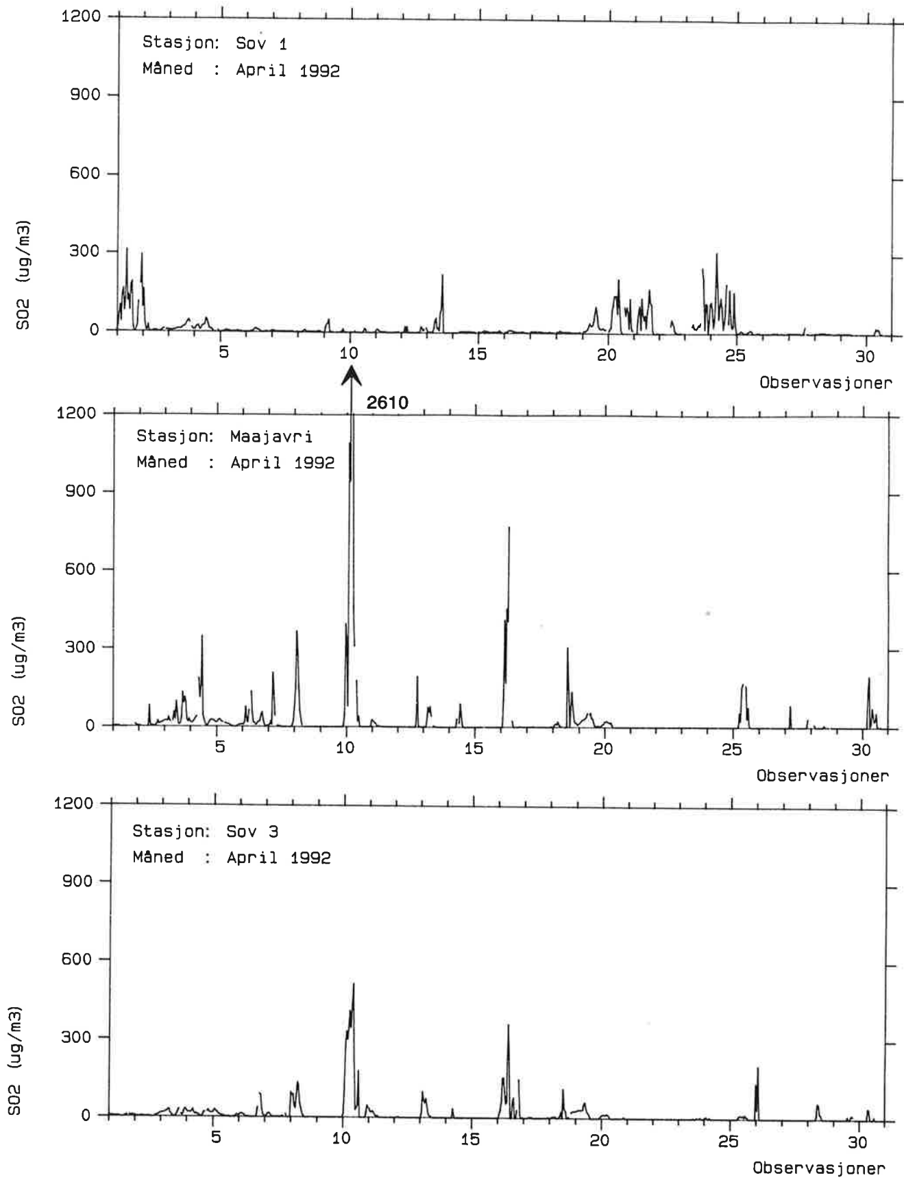
Figur 14: Timemiddelkonsentrasjoner av SO 2 i april 1992 på SOV 1, Maajavri og SOV 3 ( \mu\text{g}/\text{m}^3 ).
