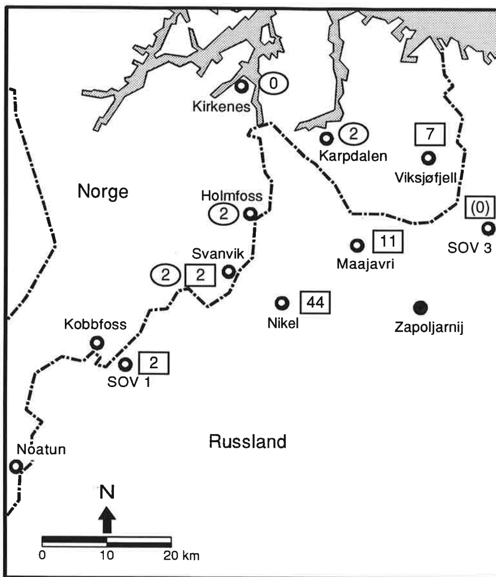
Figur 9: Antall døgnmiddelverdier av \text{SO}_2 over 90 \mu\text{g}/\text{m}^3 i perioden april-september 1992 målt med kontinuerlig registrerende prøvetakere og døgnprøvetakere . (Målingene på SOV 3 ble avsluttet 11. 6.)
