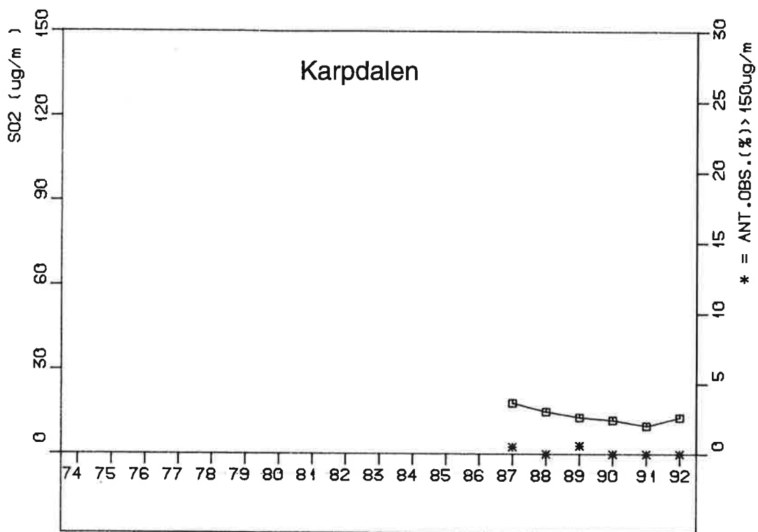
Figur 11: Sommermiddelkonsentrasjoner av SO 2 (µg/m 3 ) og frekvens av døgnmiddelverdier over 150 µg/m 3 i Holmfoss og Karpdalen.
