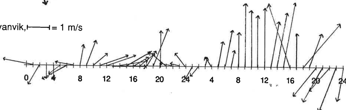
Figur 8: Timemiddelverdier av SO 2 (Viksjøfjell, Svanvik, Maajavri og Nikel), vindretning og vindstyrke (Viksjøfjell og Svanvik) 27.-28.6.1992.
