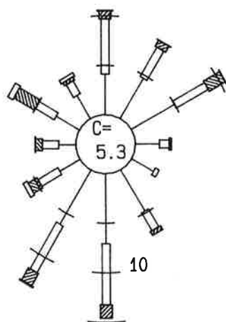
Figur 2: Vindroser for perioden april-september 1992 fra Viksjøfjell, Svanvik og Maajavri.
