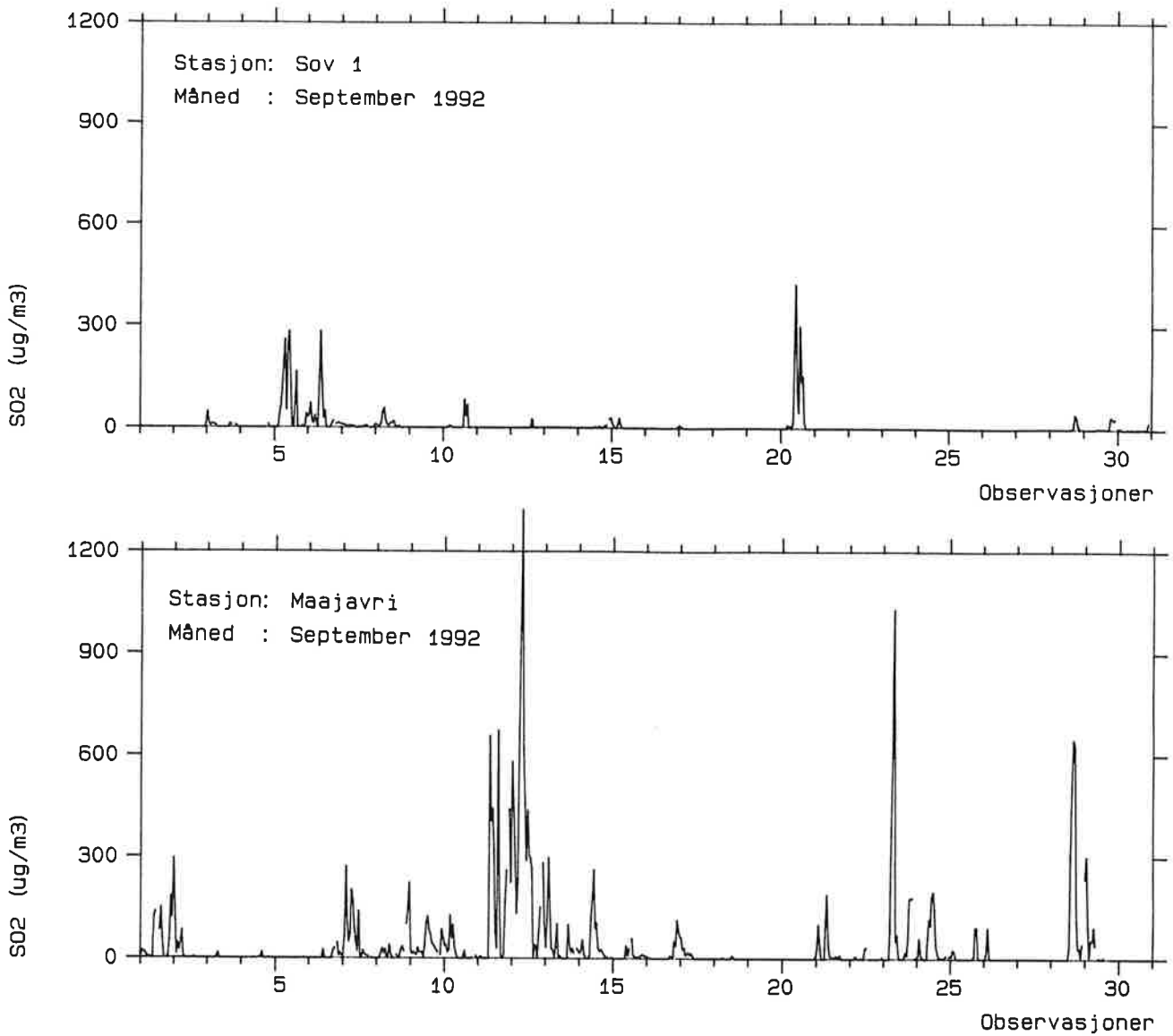
Figur 24: Middelskonsentrasjoner av SO_2 i september 1992 på SOV 1 og Maajavri ( \mu\text{g}/\text{m}^3 ).
