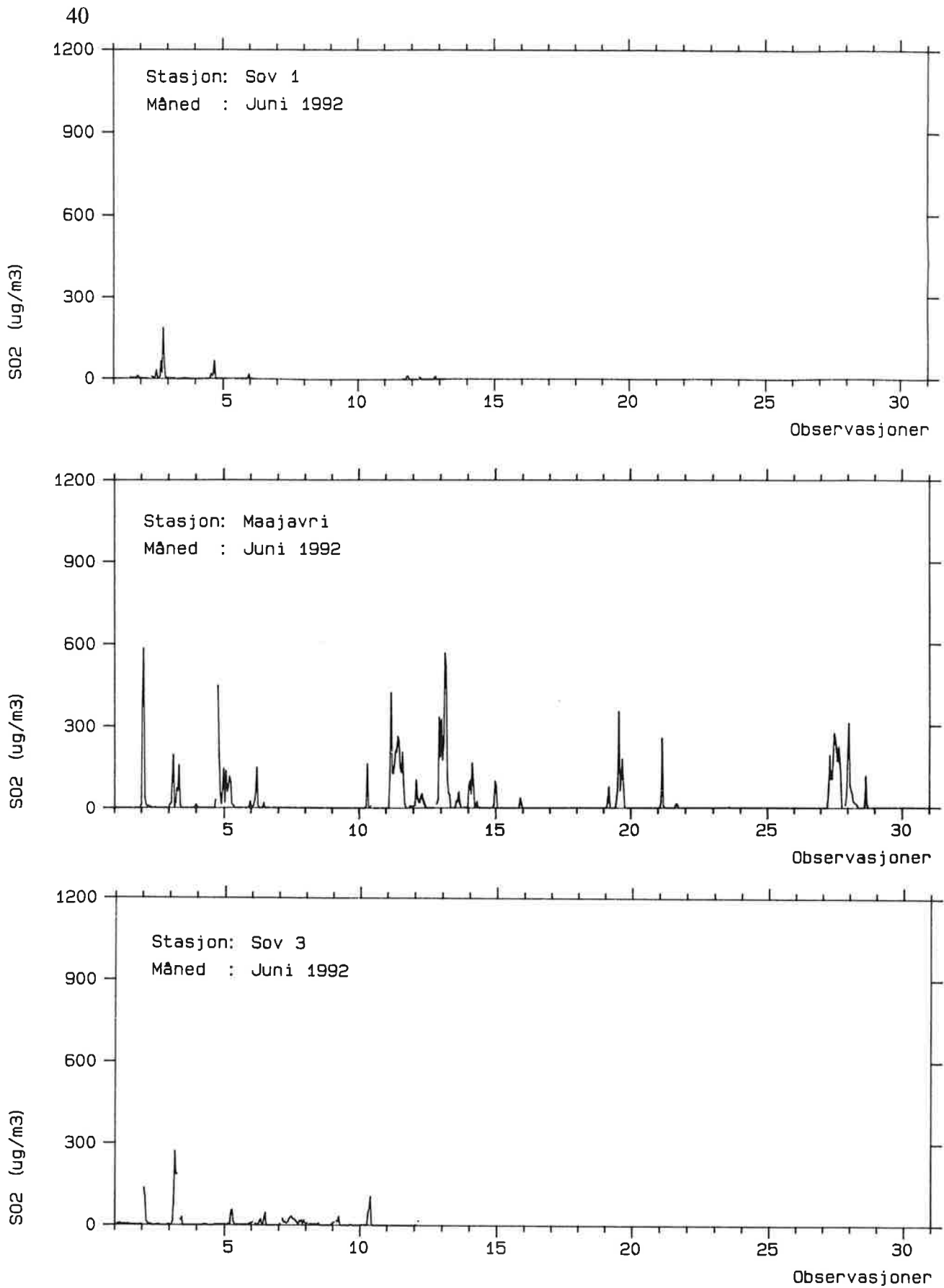
Figur 18: Timemiddelkonsentrasjoner av SO 2 i juni 1992 på SOV 1, Maajavri og SOV 3 (µg/m 3 ). Målingene på SOV 3 ble avsluttet 11.6.
