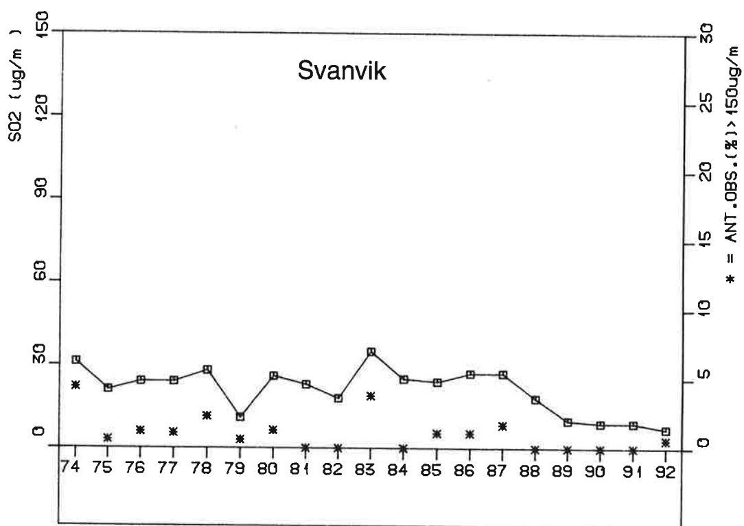
Figur 12: Sommermiddelkonsentrasjoner av SO 2 ((µg/m 3 ) og frekvens av døgnmiddelverdier over 150 µg/m 3 i Kirkenes og Svanvik.
