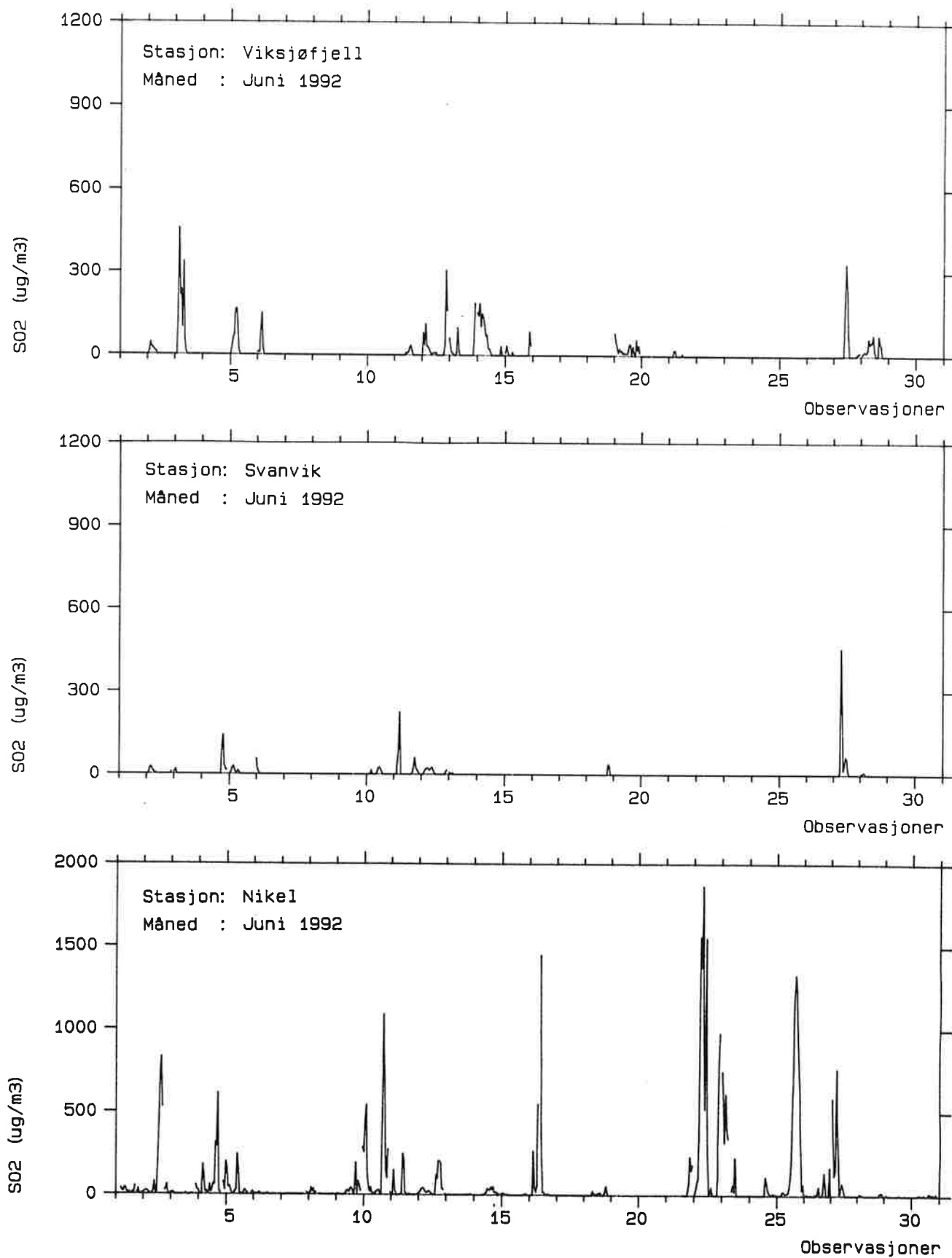
Figur 17: Timemiddelkonsentrasjoner av SO 2 i juni 1992 på Viksjøfjell, i Svanvik og i Nikel (µg/m 3 ).
