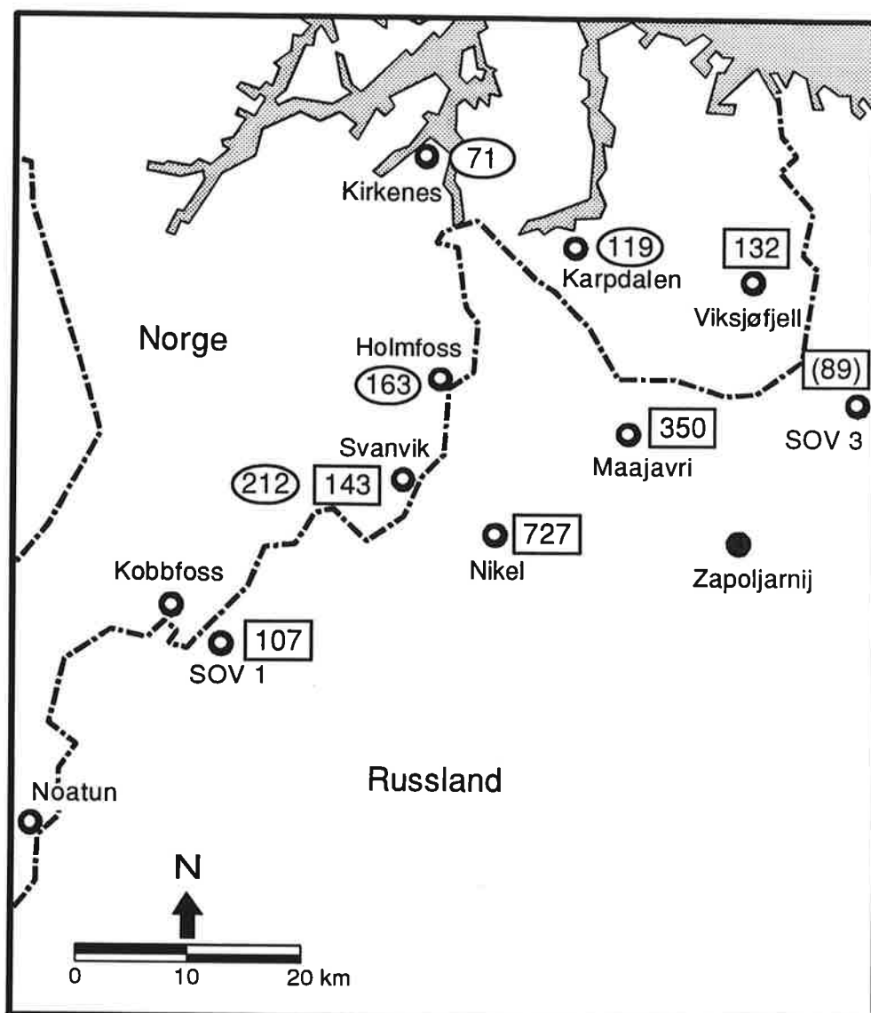
Figur 10: Maksimale døgnmiddelkonsentrasjoner av SO_2 i perioden april-september 1992 målt med kontinuerlig registrerende prøvetakere og døgnprøvetakere ( \mu g/m^3 ). (Målingene på SOV 3 ble avsluttet 11.6.)
