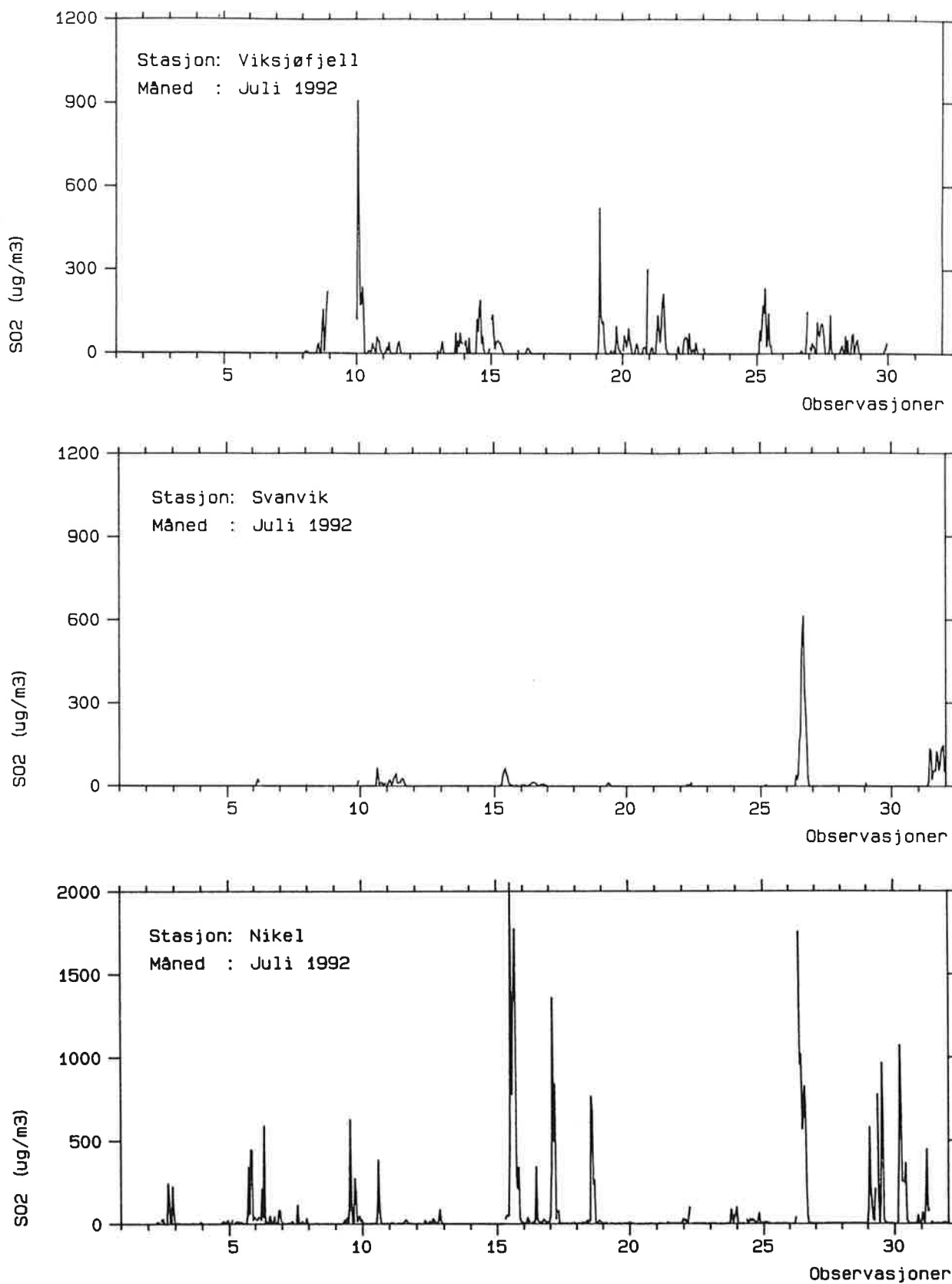
Figur 19: Timemiddelkonsentrasjoner av SO 2 i juli 1992 på på Viksjøfjell, i Svanvik og i Nikel (µg/m 3 ).
