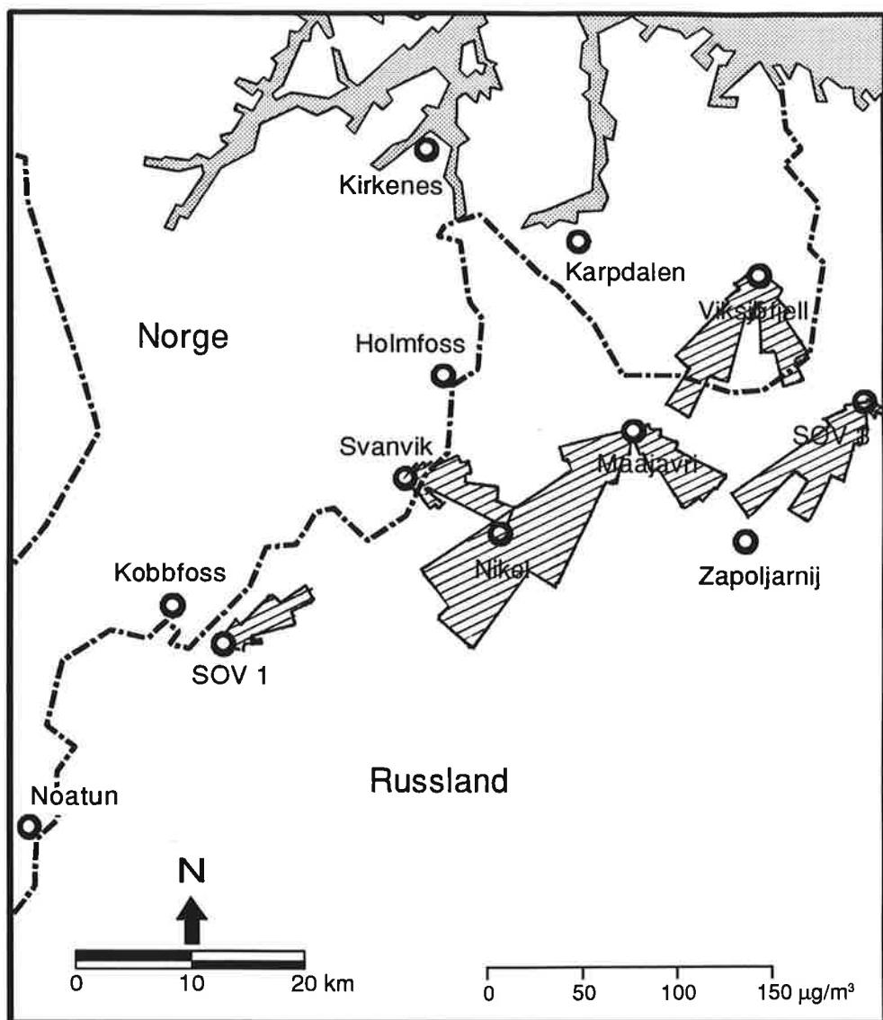
Figur 25: Middelkonsentrasjoner av SO 2 for Viksjøfjell, Svanvik, SOV 1, Maajavri og SOV 3 i 36 vindsektorer i perioden april-september 1992 (µg/m 3 ). (Målingene på SOV 3 ble avsluttet 11. juni.)
