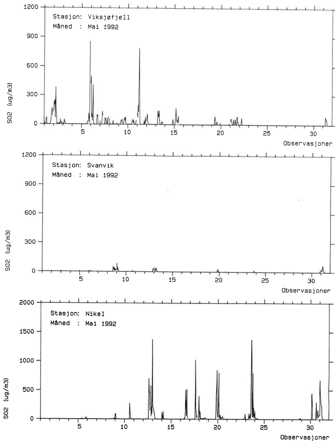
Figur 15: Timemiddelkonsentrasjoner av SO 2 i mai 1992 på Viksjøfjell, i Svanvik og i Nikel (µg/m 3 ).
