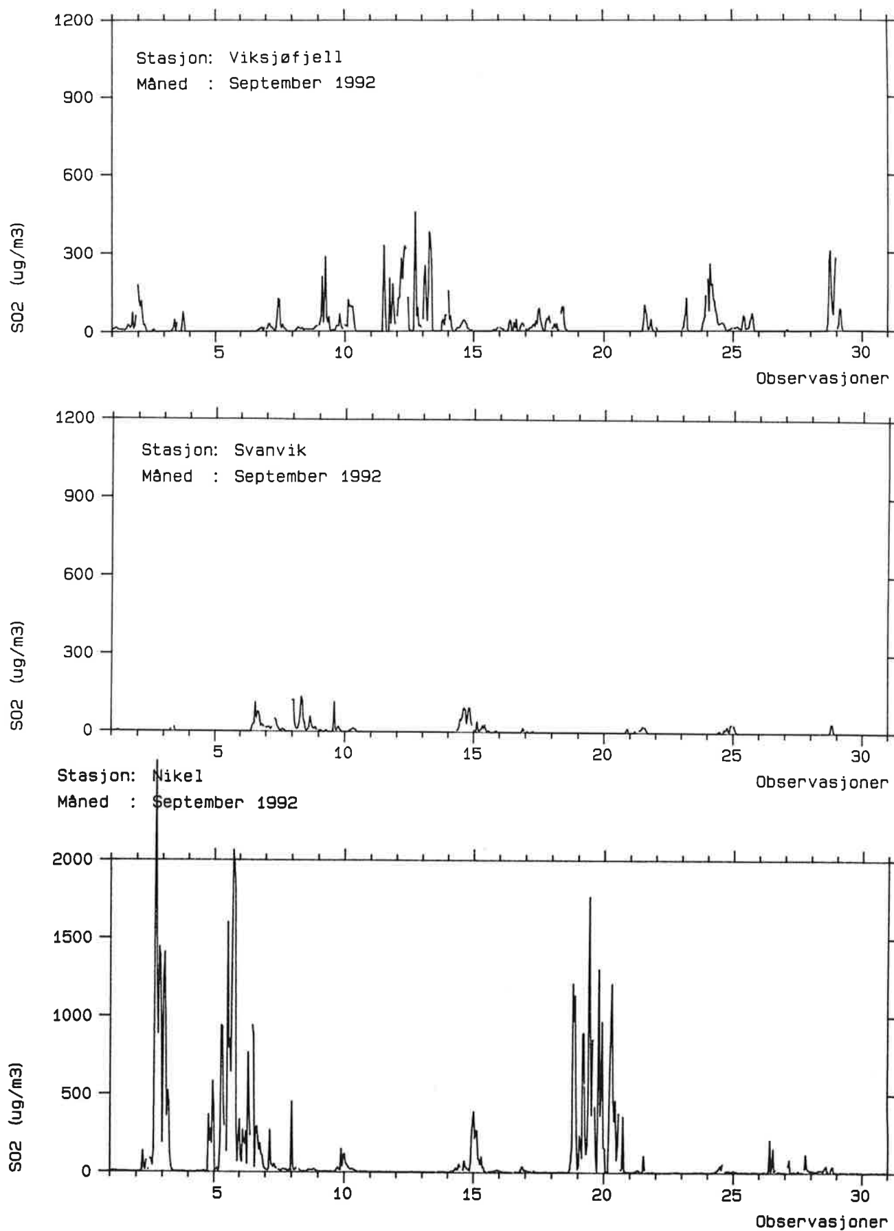
Figur 23: Timemiddelkonsentrasjoner av SO 2 i september 1992 på Viksjøfjell, i Svanvik og i Nikel (µg/m 3 ).
