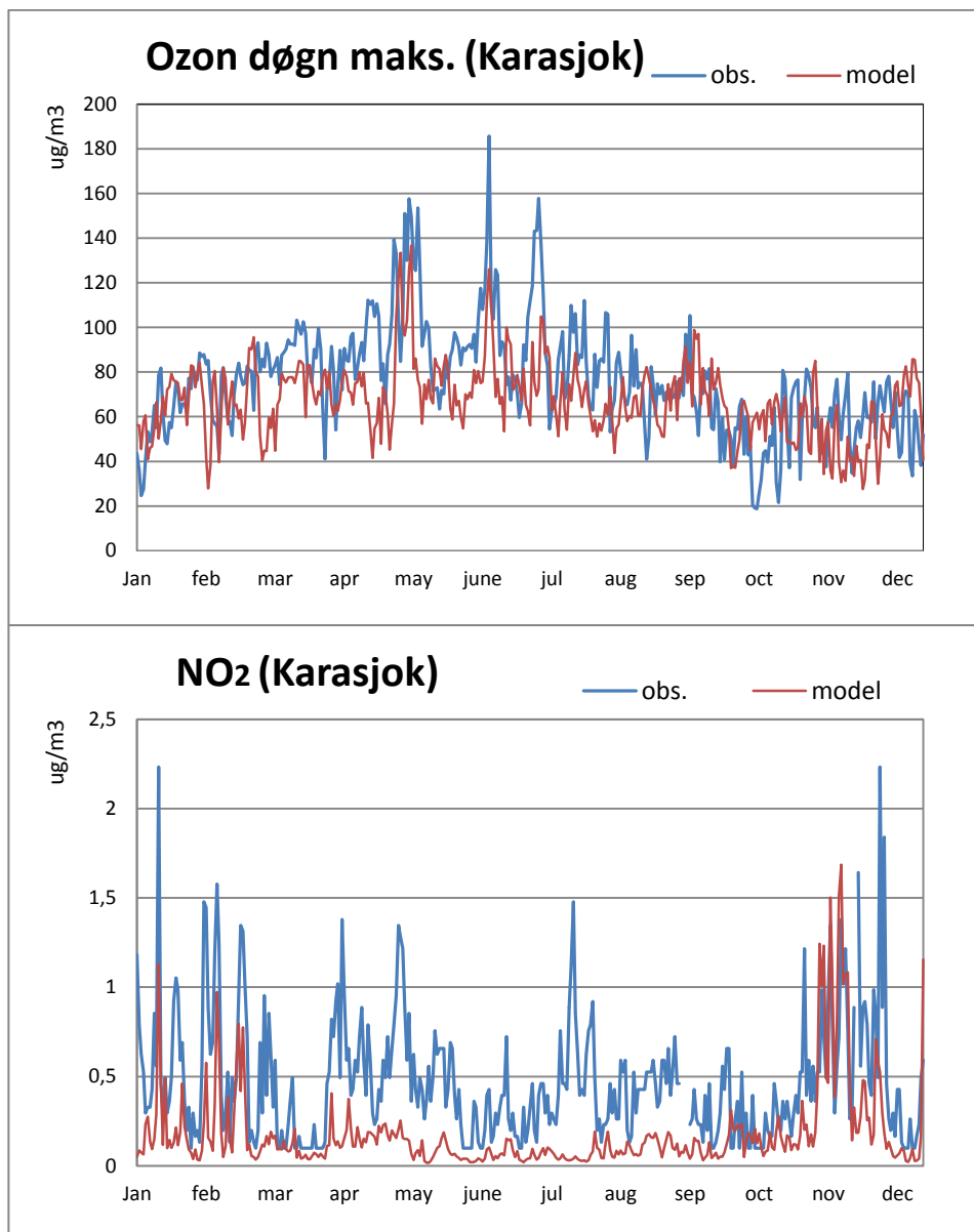
Figur 6.3: Modellerte og målte verdier av døgnlign maksimal ozonkonsentrasjon og døgnmiddel av NO 2 i 2006 på Zeppelin-stasjonen (Ny-Ålesund) og Karasjok. Enhet: ug/m 3 .
