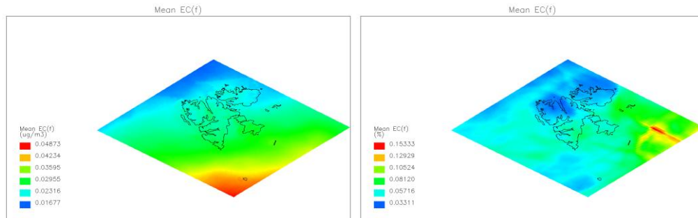
Figur 6.10: Beregnet årsmiddelmiddelkonsentrasjon i finfraksjonen av BC på Spitsbergen for bakgrunns-situasjonen (venstre) og den relative økningen pga petroleumsutslippene (høyre). Enheter: \mu\text{g}/\text{m}^3 og %.
