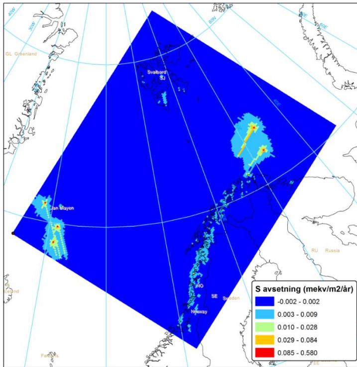
Figur 8.7: Beregnet avsetning av S på grunn av utlipp fra petroleumsvirksomhet ved Jan Mayen og i Barentshavet.
