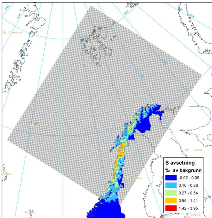
Figur 8.8: Beregnet S-avsetning som ‰ (promille) av bakgrunnsavsetning på grunn av utlipp fra petroleumsvirksomhet ved Jan Mayen og i Barentshavet.
