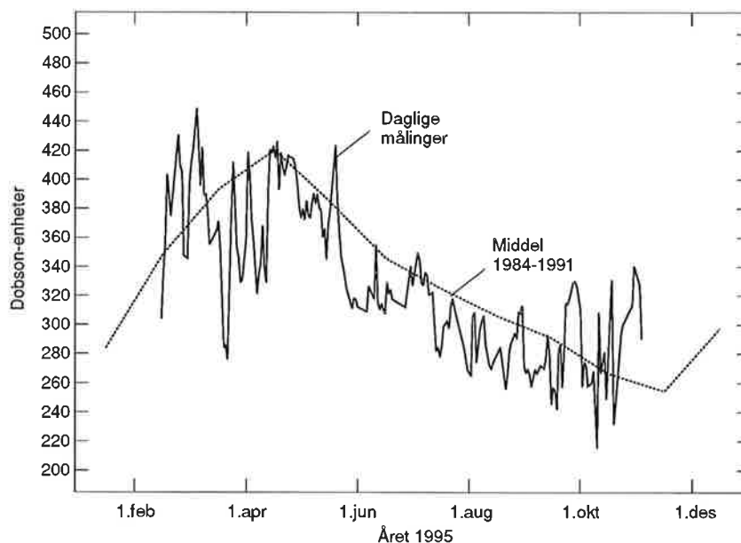
Figur 2: Daglige ozonverdier målt med Dobson- og Brewer-instrumentene ved Universitetet i Tromsø i 1995. Den stiplede kurven er månedsmidlene fra 1984 til 1991.
