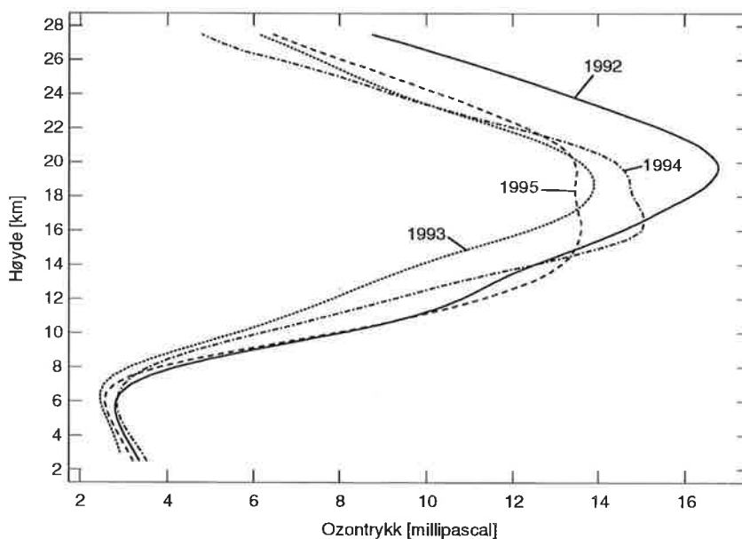
Figur 10: Midlere høydefordeling av ozon for januar-april for årene 1992 til 1995 over Bjørnøya.
