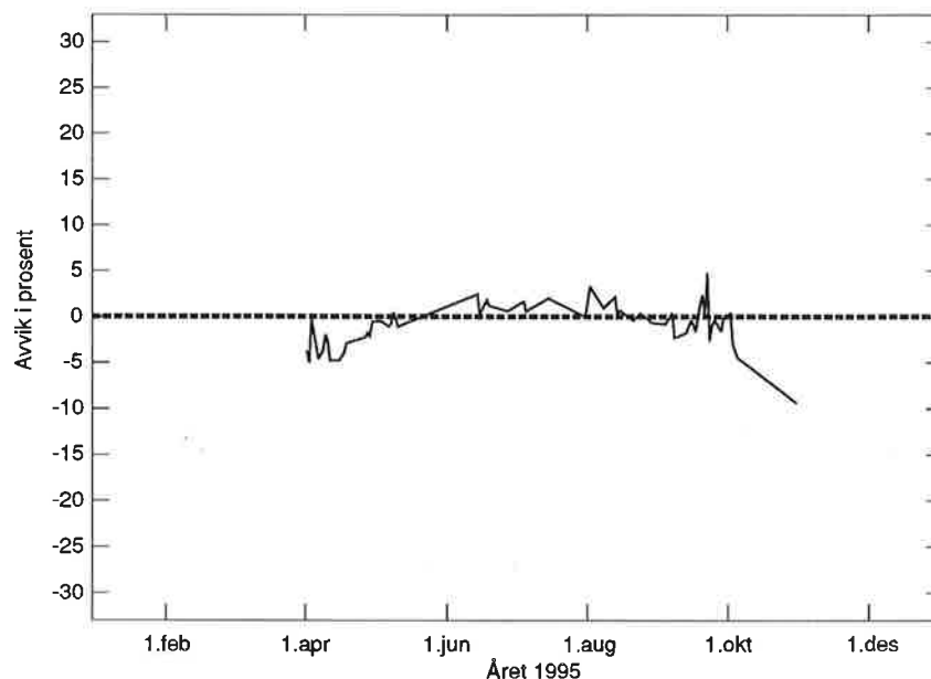
Figur 20: Sammenligning mellom ozonmåliner utført med Dobson- og Brewer-instrumentet for Tromsø i 1995, 100 \cdot (\text{Dobson} - \text{Brewer}) / \text{Dobson} .
