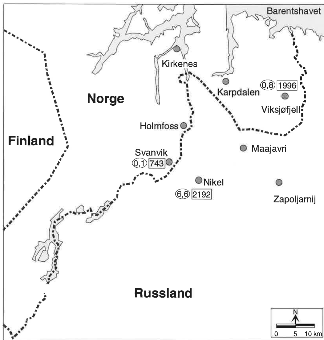
Figur 16: Maksimale timemiddelverdier av SO 2 (µg/m 3 ) og prosent av tiden med timemiddelverdier over 350 µg/m 3 i perioden april-september 1994.
