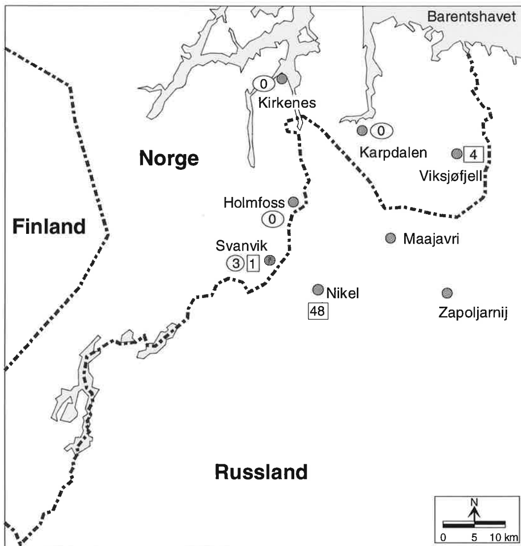
Figur 6: Antall døgnmiddelverdier av \text{SO}_2 over 90 \mu\text{g}/\text{m}^3 i perioden april-september 1994 målt med kontinuerlig registrerende prøvetakere og døgnsprøvetakere .
