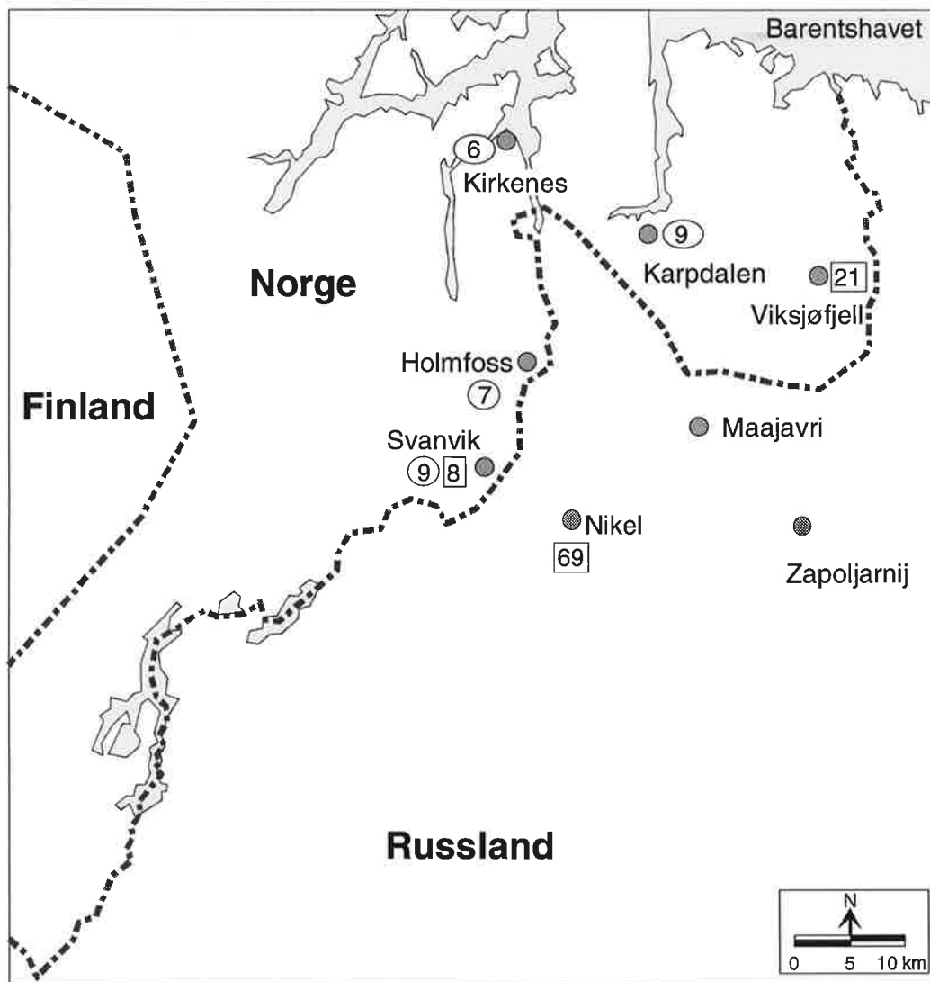
Figur 3: Middelkonsentrasjoner av \text{SO}_2 ( \mu\text{g}/\text{m}^3 ) i perioden april-september 1994 målt med kontinuerlig registrerende prøvetakere og døgnsprøvetakere .
