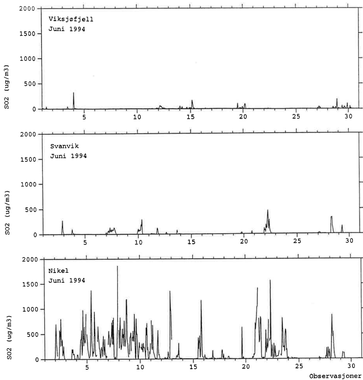
Figur 12: Timemiddelkonsentrasjoner av SO 2 i juni 1994 fra Viksjøfjell, Svanvik og Nikel (µg/m 3 ).
