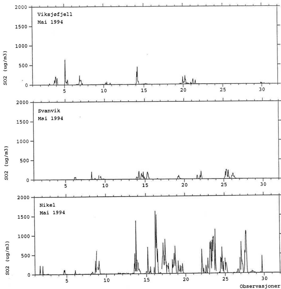
Figur 11: Timemiddelkonsentrasjoner av SO 2 i mai 1994 fra Viksjøfjell, Svanvik og Nikel ( \mu\text{g}/\text{m}^3 ).
