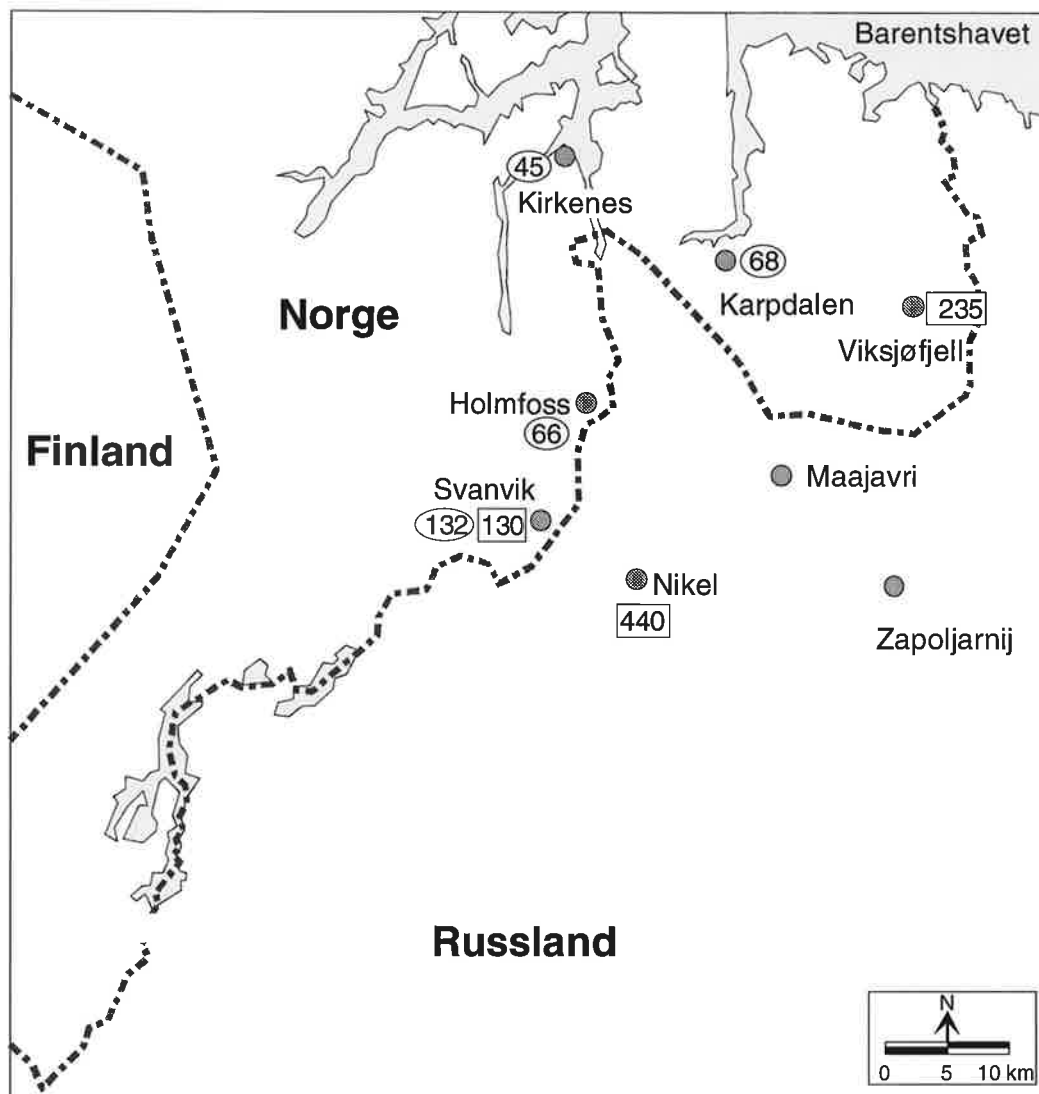
Figur7: Maksimale døgnmiddelkonsentrasjoner av SO 2 (µg/m 3 ) i perioden april-september 1994 målt med kontinuerlig registrerende prøvetakere og døgnprøvetakere .
