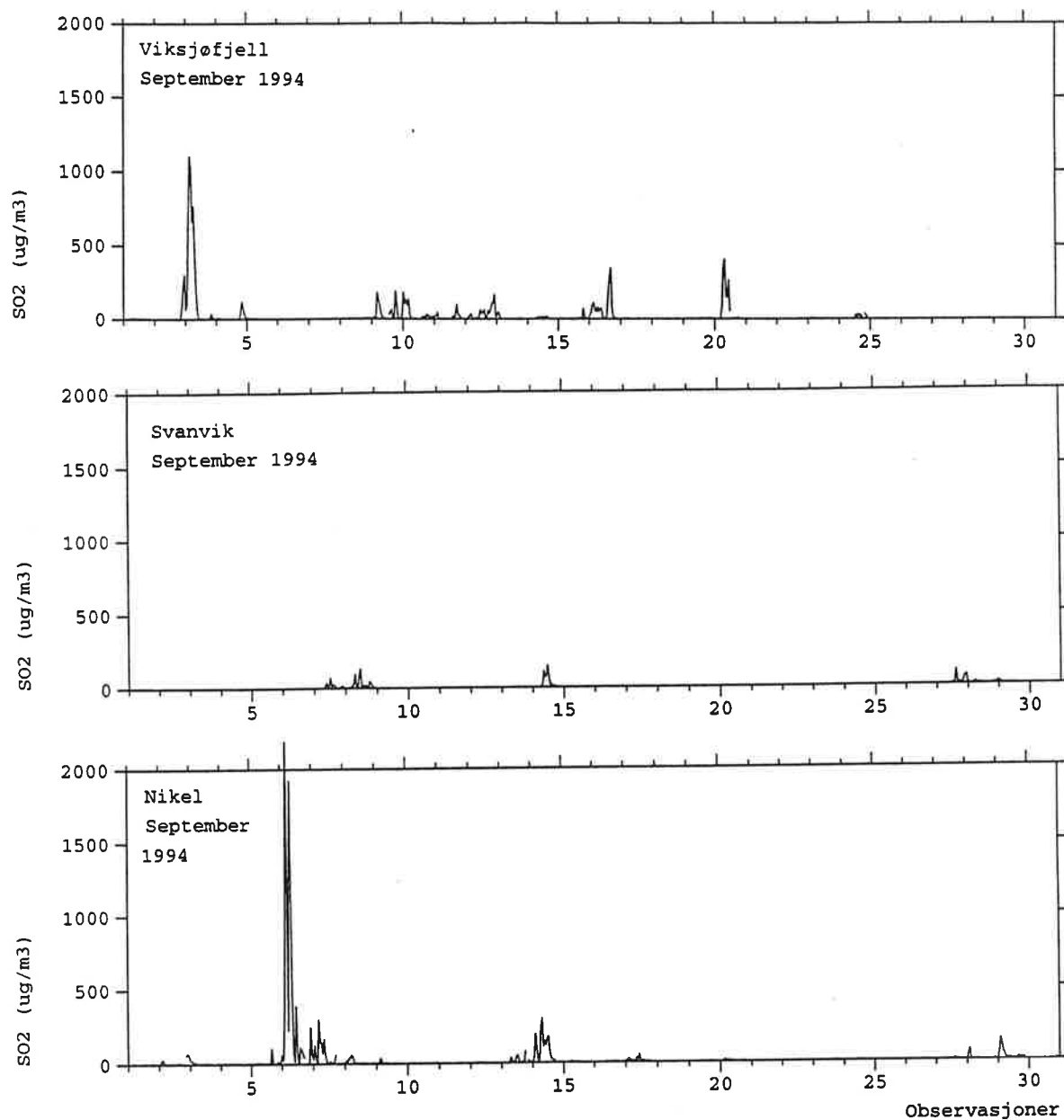
Figur 15: Timemiddelkonsentrasjoner av \text{SO}_2 i september 1994 fra Viksjøfjell, Svanvik og Nikel ( \mu\text{g}/\text{m}^3 ).
