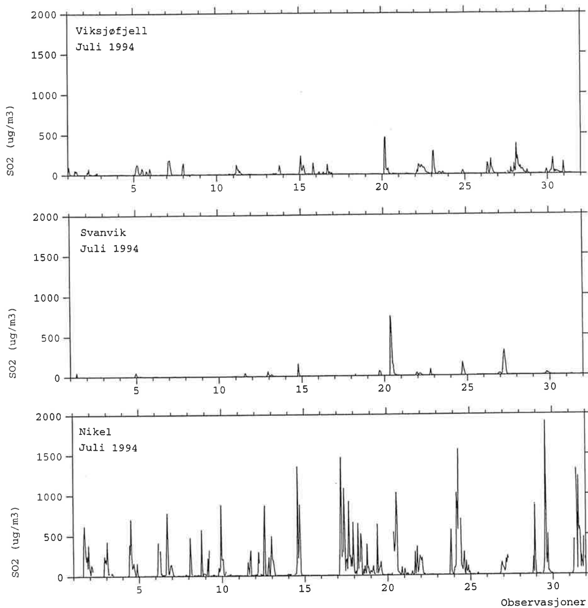
Figur 13: Timemiddelkonsentrasjoner av SO 2 i juli 1994 fra Viksjøfjell, Svanvik og Nikel (µg/m 3 ).
