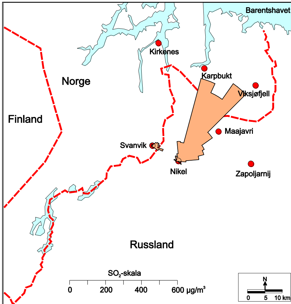
Figur 4: Middelskonsentrasjoner av SO 2 i Svanvik og Nikel i perioden oktober 2006-mars 2007 (µg/m 3 ). Figuren viser middelskonsentrasjoner av SO 2 for hver av 36 10 o -vindsektorer. Begge stasjonene er mest belastet når det blåser fra smelteverket i Nikel.
